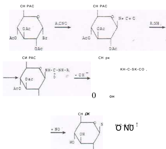
R = алкил, хлорэтил Схема 1
